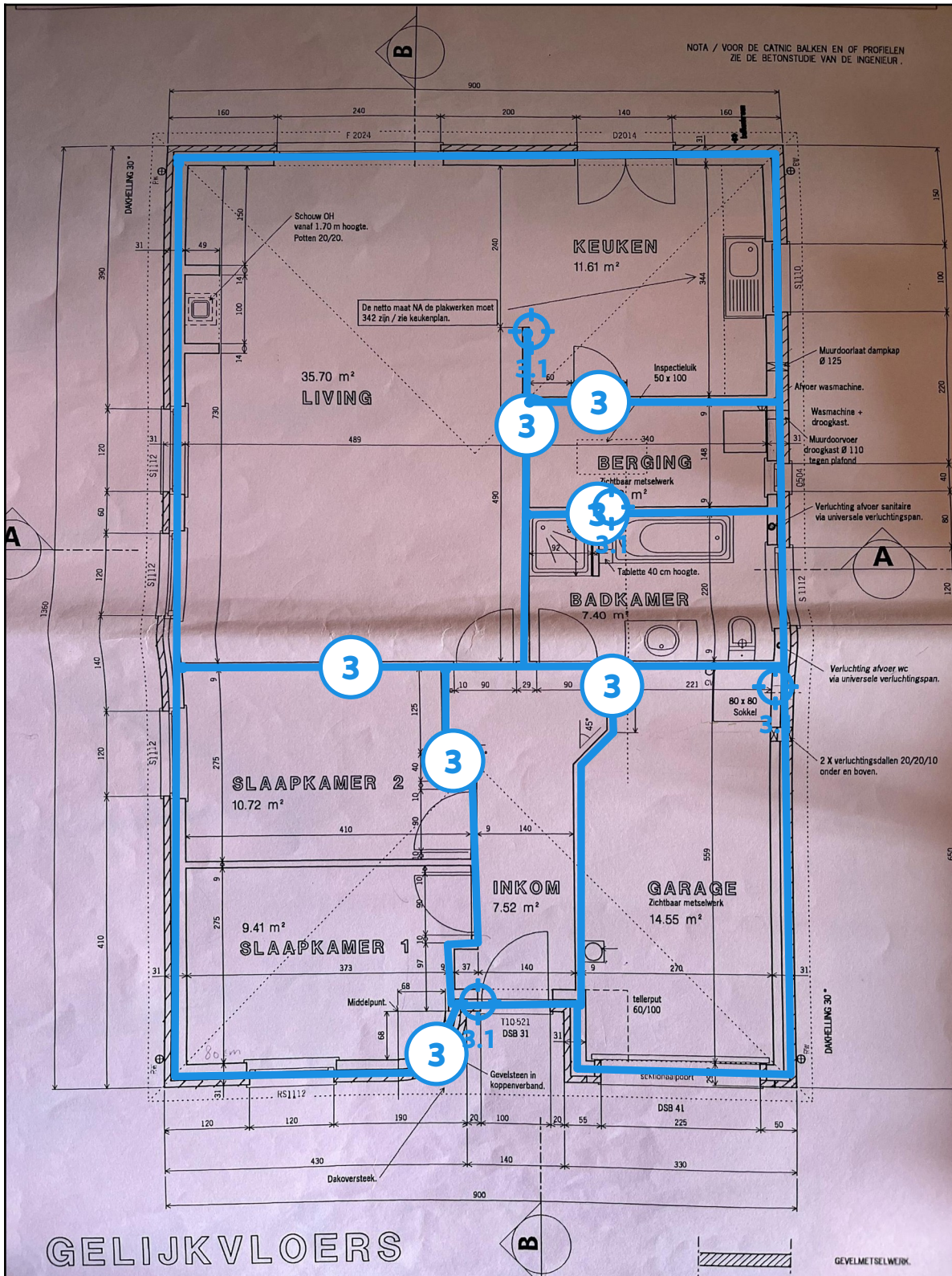
Legende van plan 1.1: Gelijkvloers - Pleisterwerk
